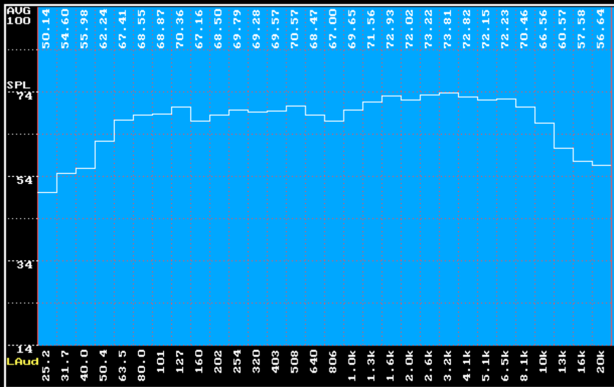
Réponse en fréquence en 1/3 octave
